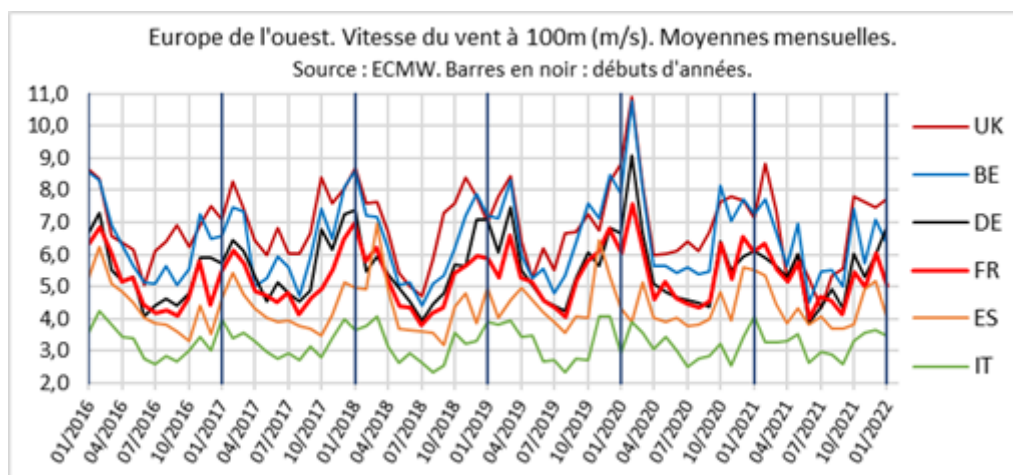
Vitesse moyenne du vent à 100 mètres (en m/s) en Europe de l'ouest
